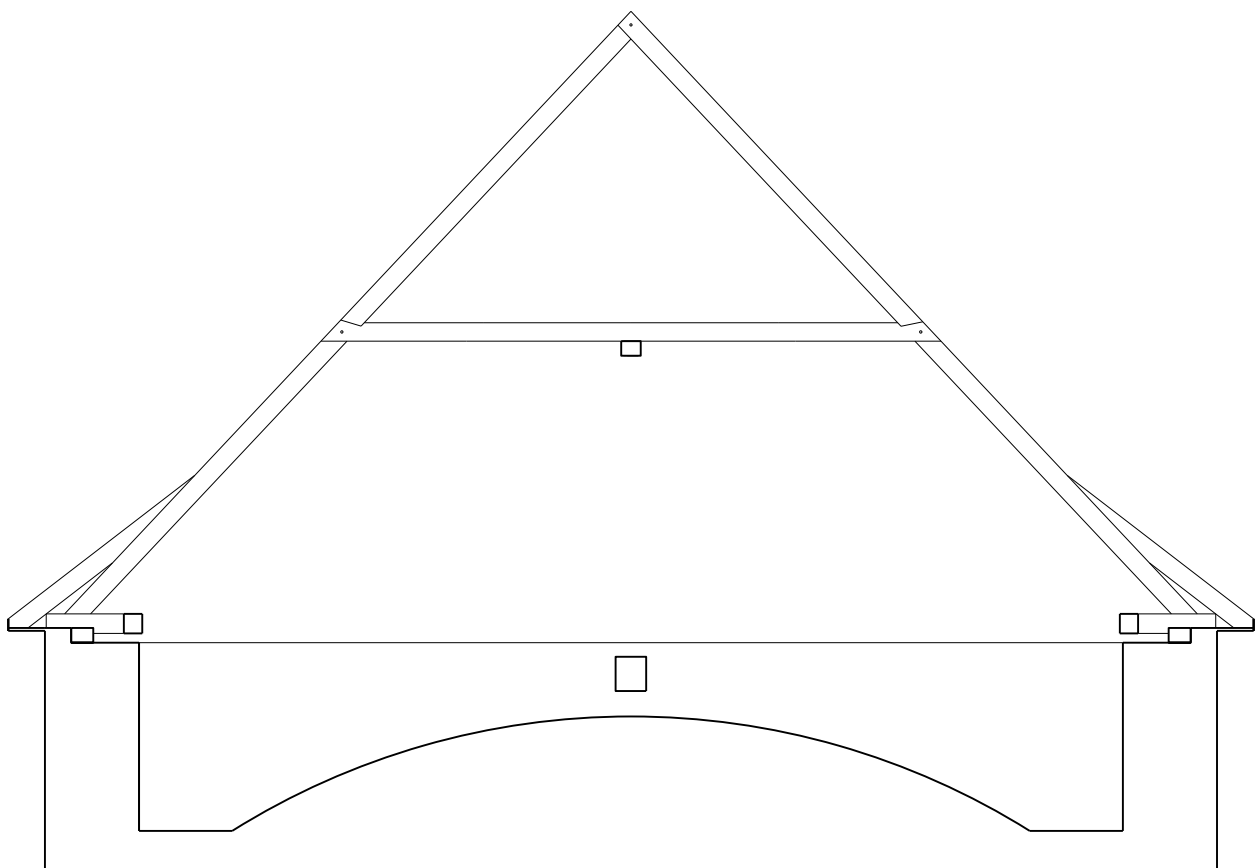
LOŤ KOSTOLA - plná vřzba
